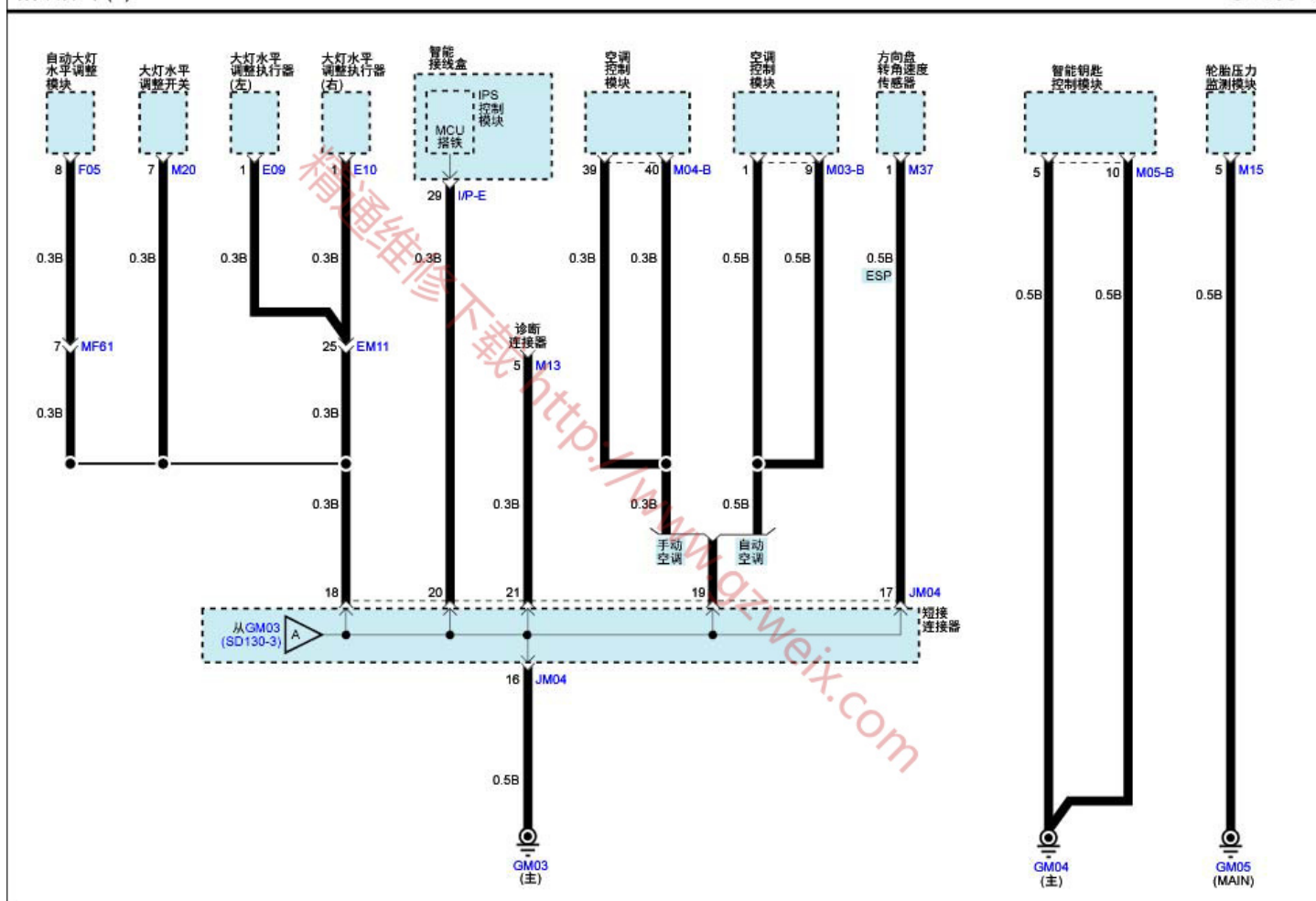
搭铁分布(4)
